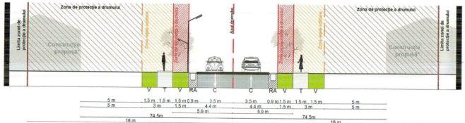
Profilul străzii drum comun și alte drumuri secundare 1) Titlu nr. 1/2013, în baza cărții tehnice de proiectare nr. 1/2013 2) în baza CNAIR sau, după caz a serviciilor publice deconcentrate ale acestuia
