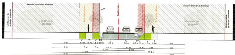
Profilul străzii situația propusă - Drumul Județean 108 D 1) Titlu nr. 1/2013, în baza cărții tehnice de proiectare nr. 1/2013 2) în baza CNAIR sau, după caz a serviciilor publice deconcentrate ale acestuia
